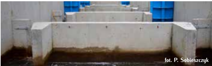
Przepławka dwuszczelinowa przy stopniu w km 108+080 Wisłoki w miejscowości Jasto.
