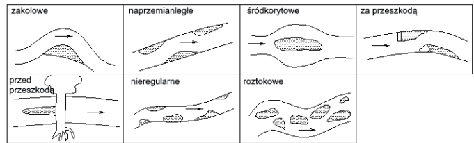
Typy łach korytowych (za: Stream Hydrology. An Introduction for Ecologists | Gordon et al. Wiley and Sons 1992)
